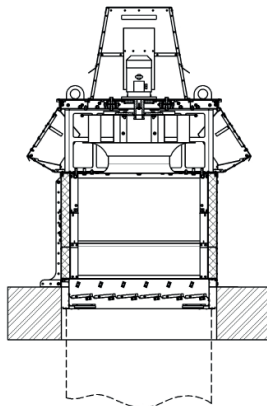
Клапан снаружи
