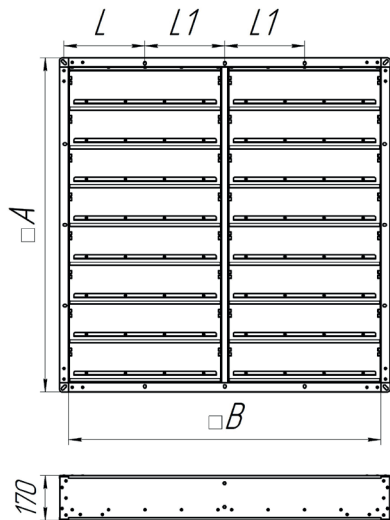
Внешний обратный клапан
