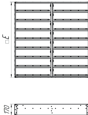
Внутренний обратный клапан
