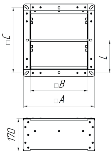
Внешний обратный клапан
